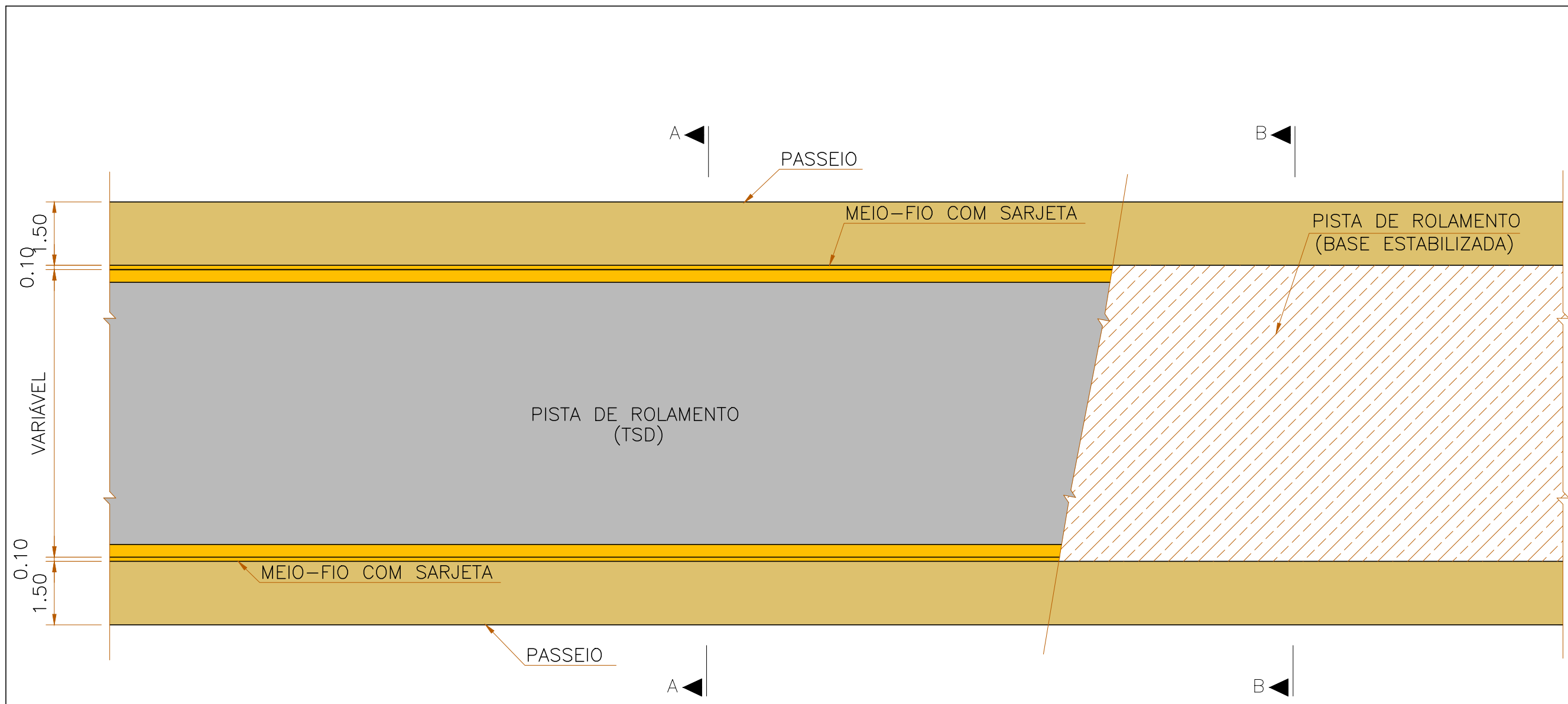
PAVIMENTAÇÃO TÍPICA – 05 PLANTA ESC. 1:100
